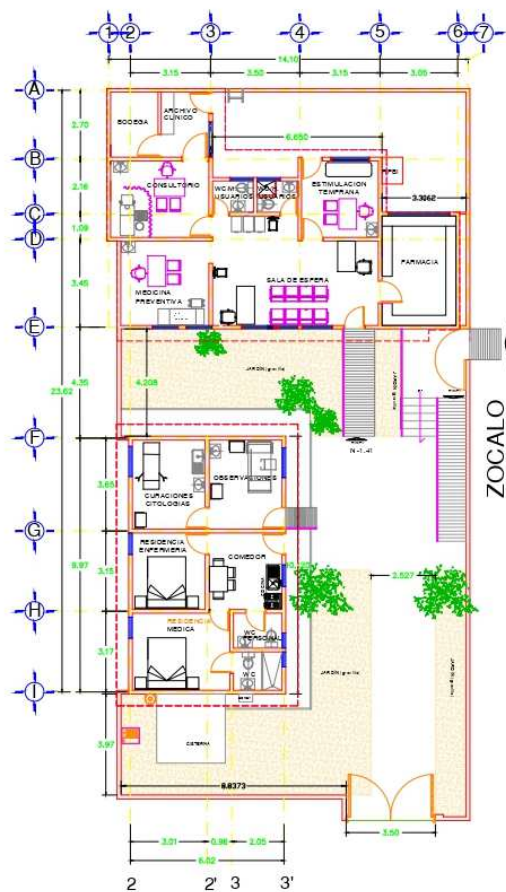
PLANTA ARQUITECTÓNICA
