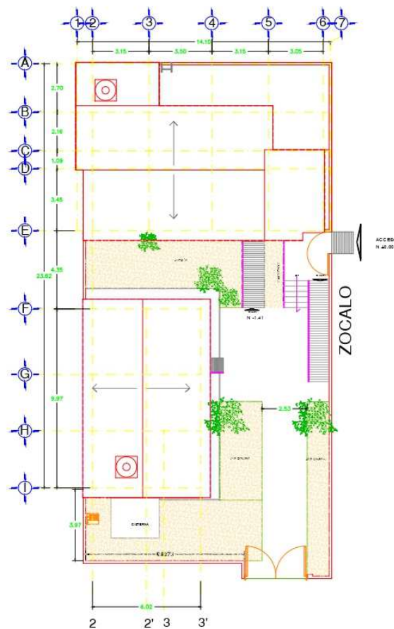
PLANTA AZOTEA
