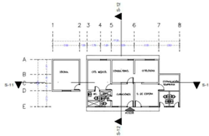
CS Huitchila: Plano arquitectónico
