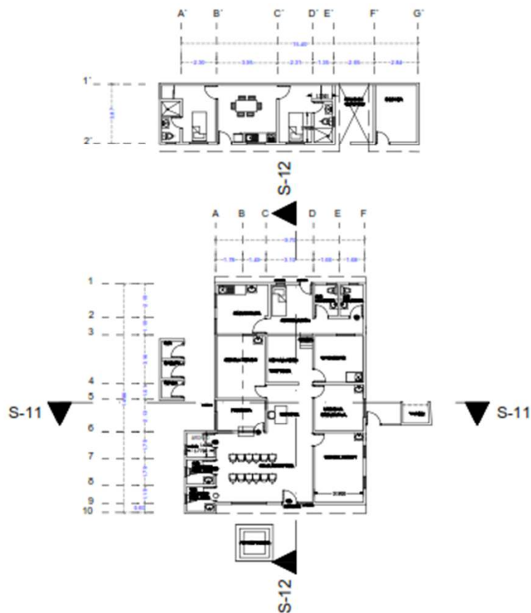
CS Atlacahualoya: Plano arquitectónico
